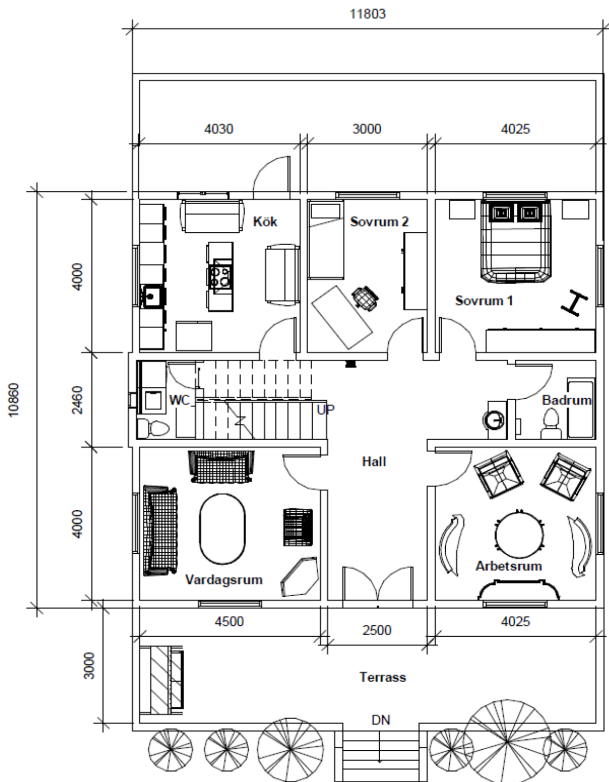
Level 1 1 : 100
