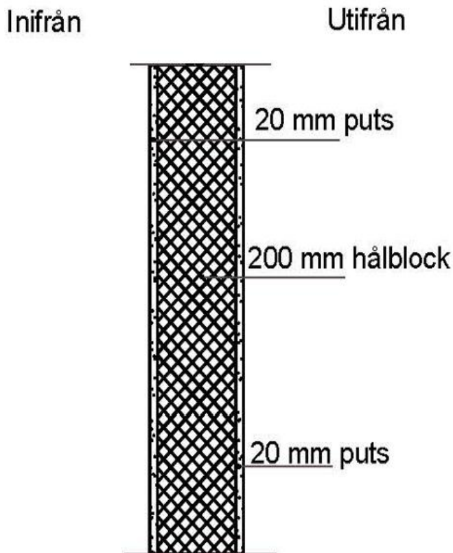
Figur 4.4 Yttervägg konstruktion
