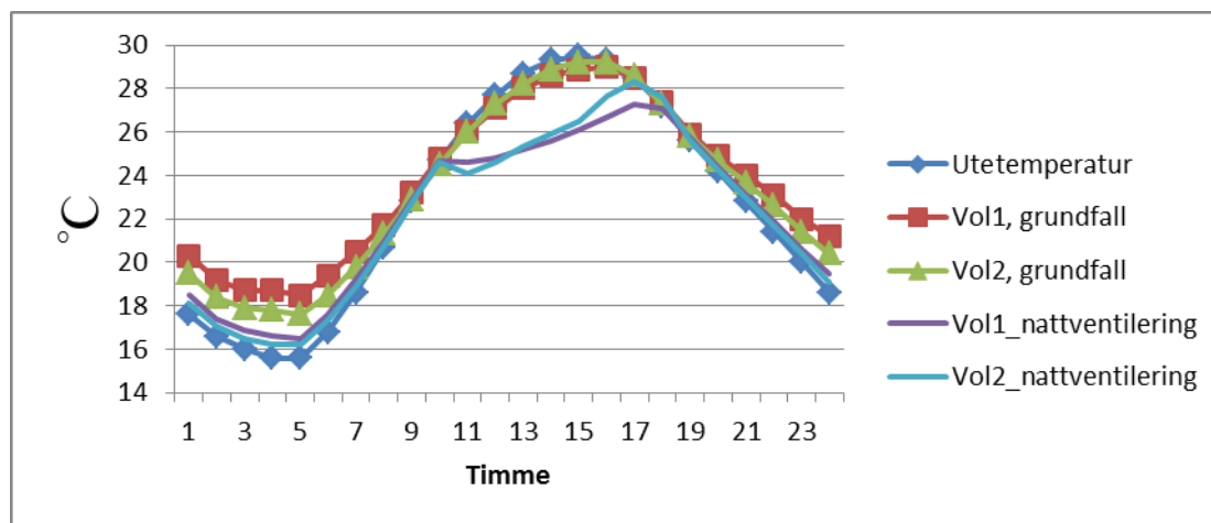
Figur 6.4 temperaturvariation vid nattventilering mellan kl.18-11
