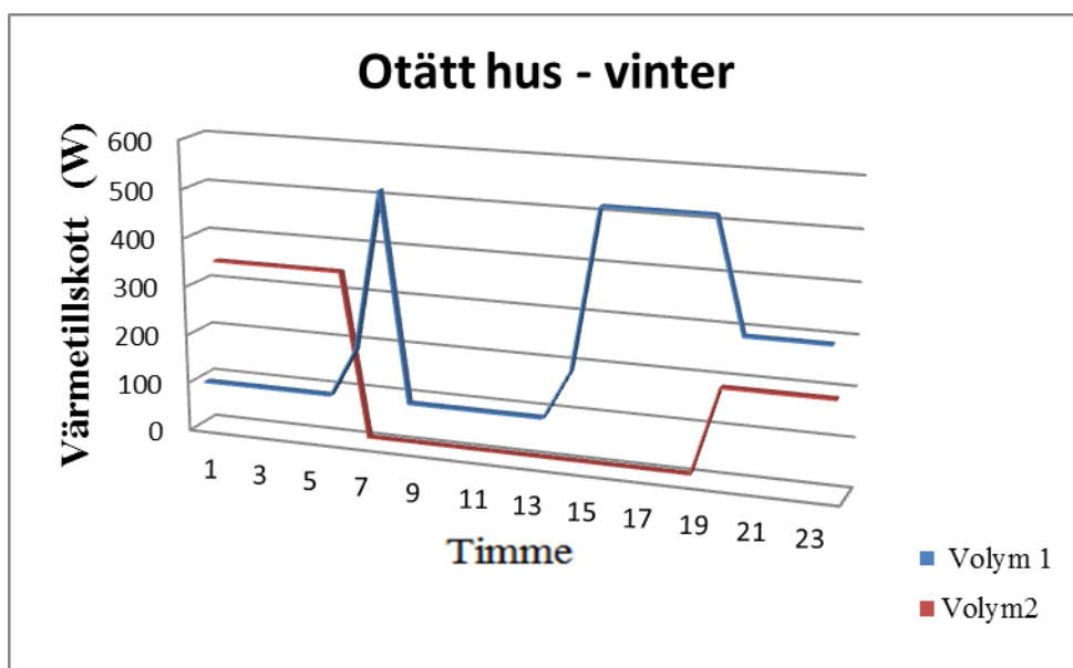
Figur 5.5 Antagna värmeförlustvärden i huset under vintern
